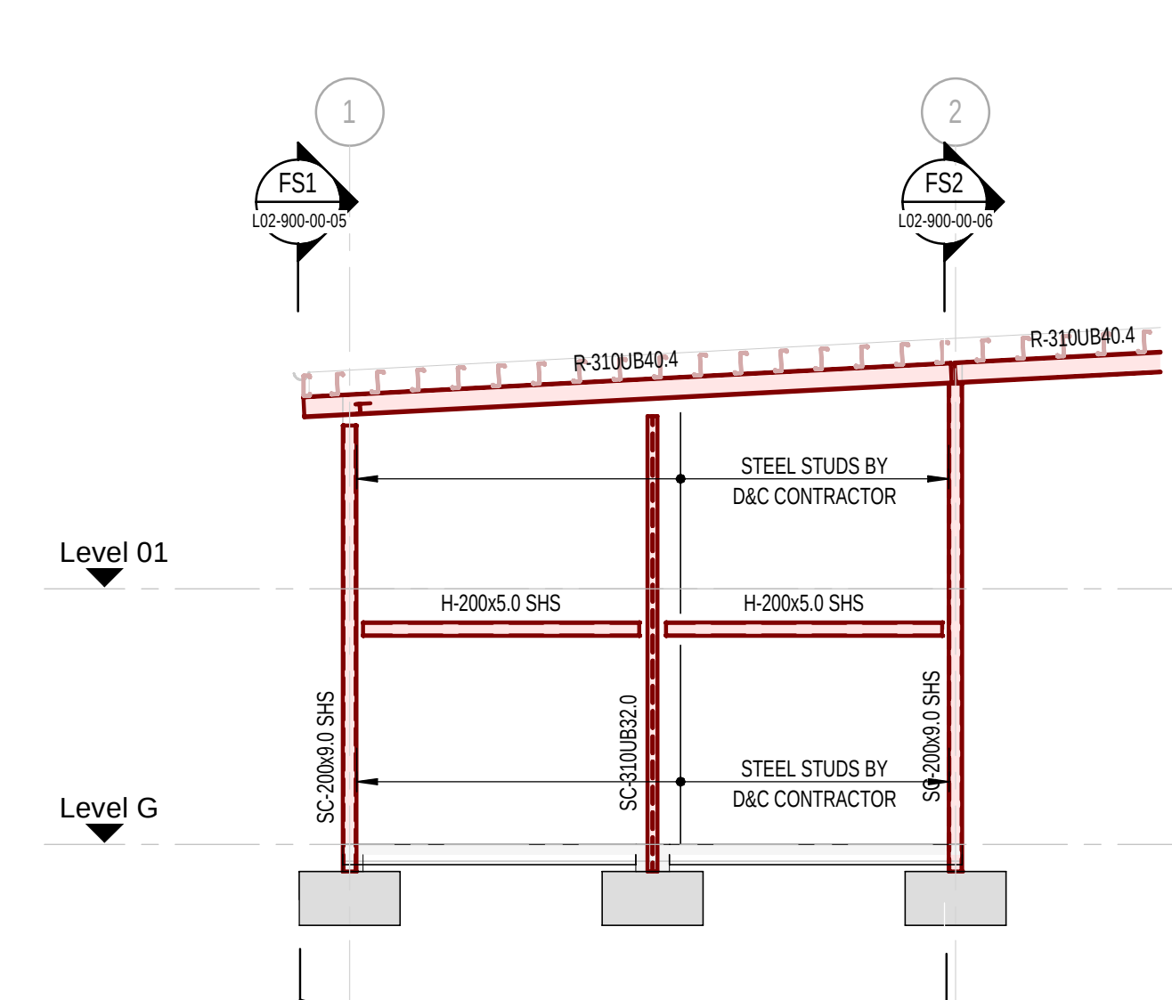
SECTION FS17 SCALE 1 : 100 L02-510-00-02
